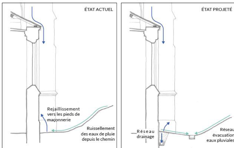
À gauche, schéma des dispositions actuelles des sols au nord de l'église. À droite, schémas des dispositions projetées du réseau d'assainissement, du réseau de drainage et du réaménagement des sols (documents NASCA).
